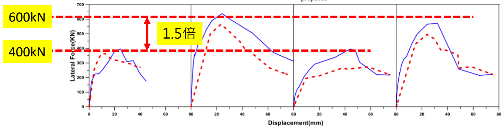
CFRP補強含開口磚牆側力與位移關係分析結果比較
