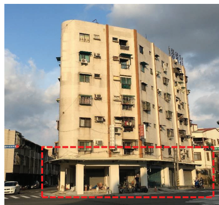
補強後
