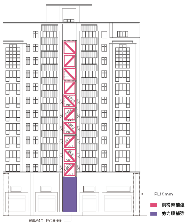
補強立面圖
