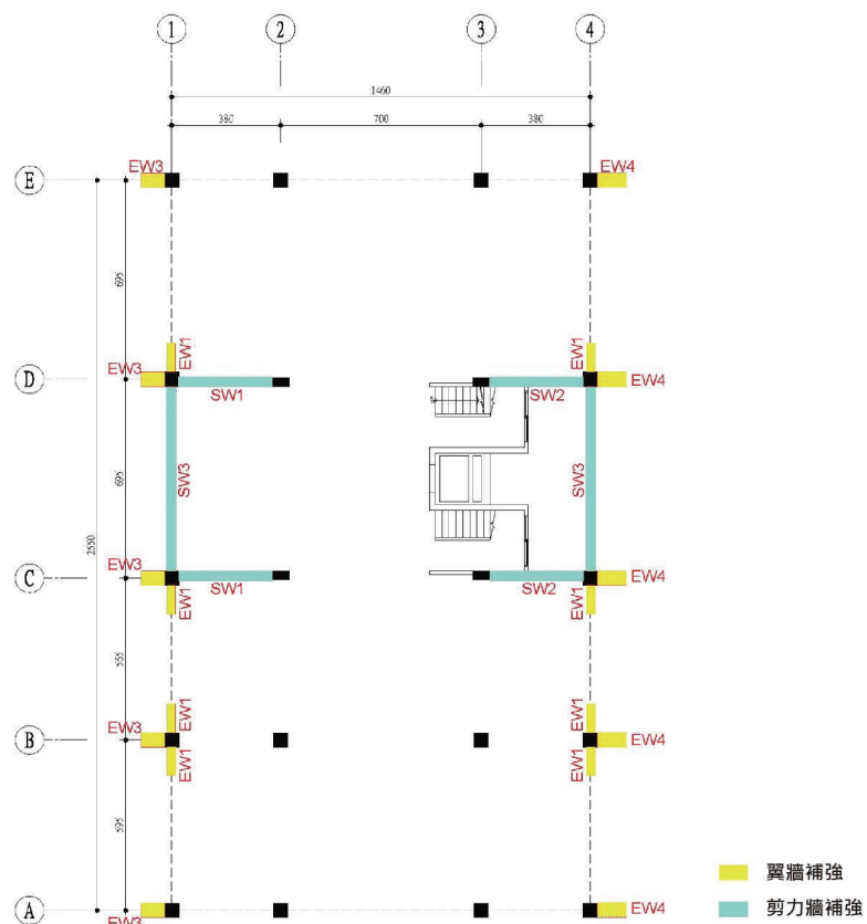
補強位置平面圖
