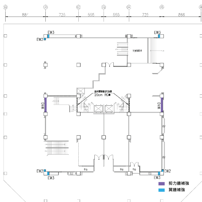
補強平面圖
