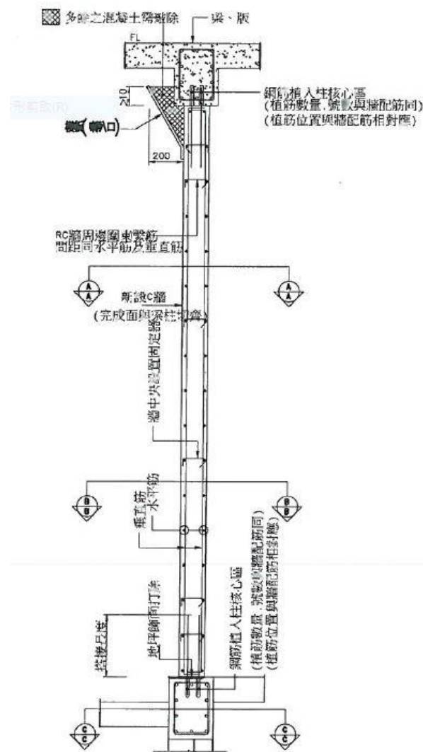
RCW1-1 立面圖
