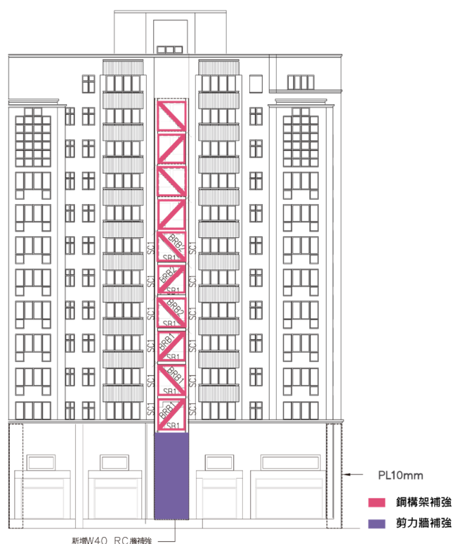
補強立面圖
