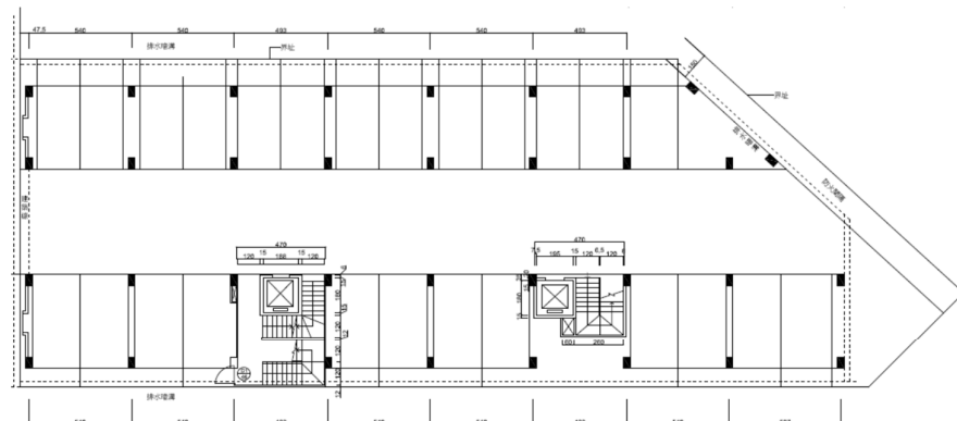
原始1F建築平面圖
