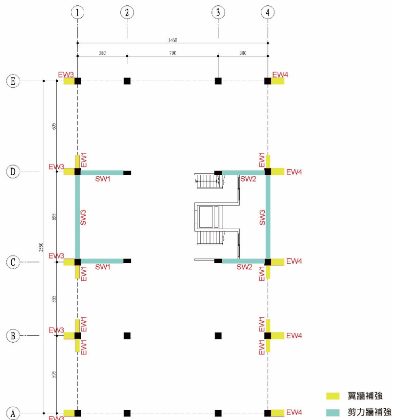
補強位置平面圖
