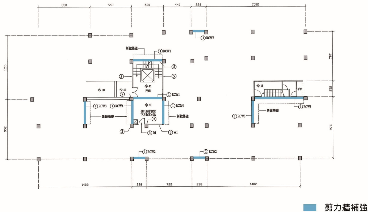
補強位置平面圖
