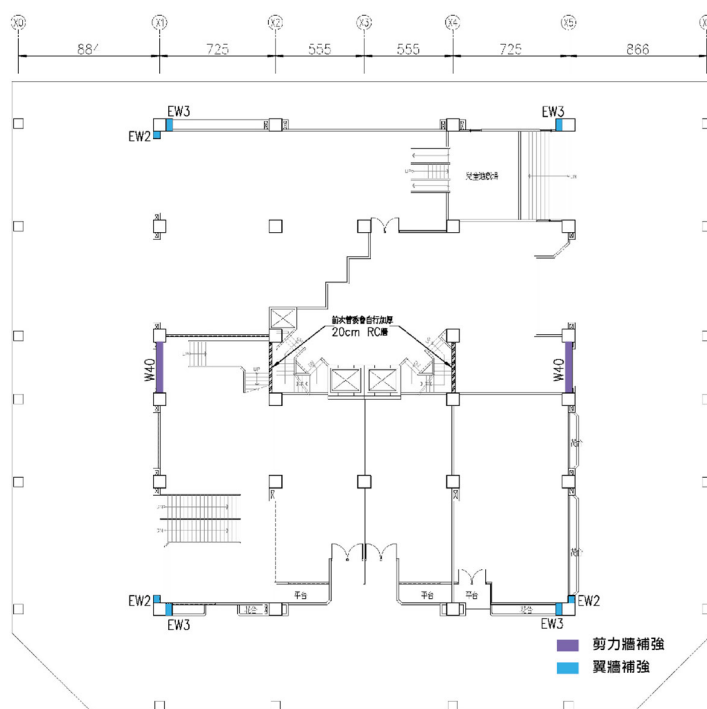
補強平面圖
