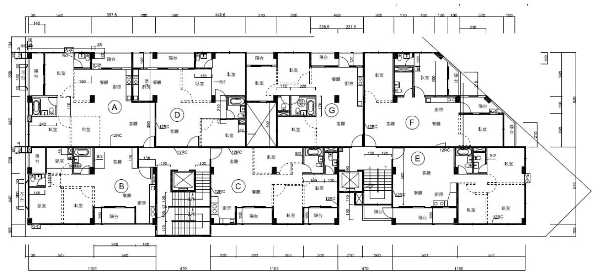
原始2~5F建築平面圖
