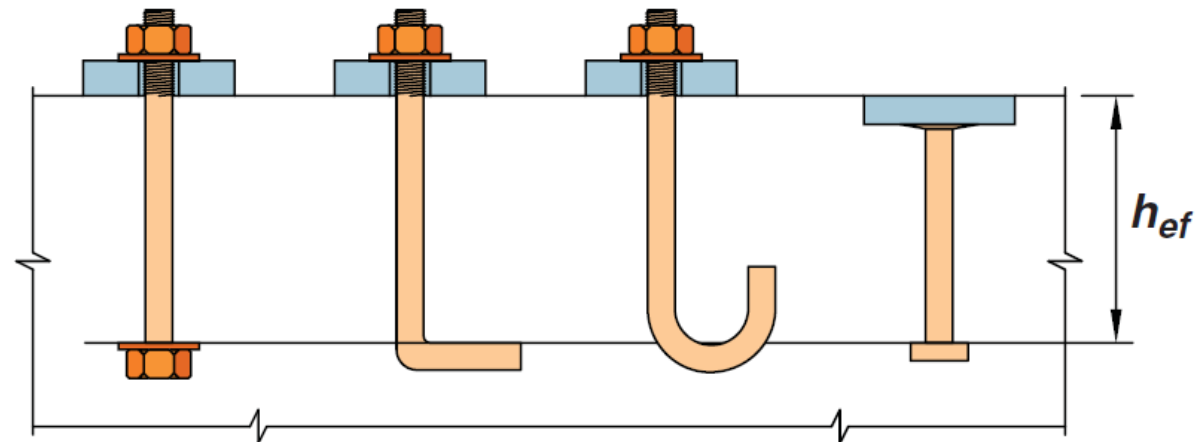
預埋式錨栓 (a) 六角頭螺栓含墊片 (b) L型錨栓 (c) J形錨栓 (d) 焊接剪力釘
