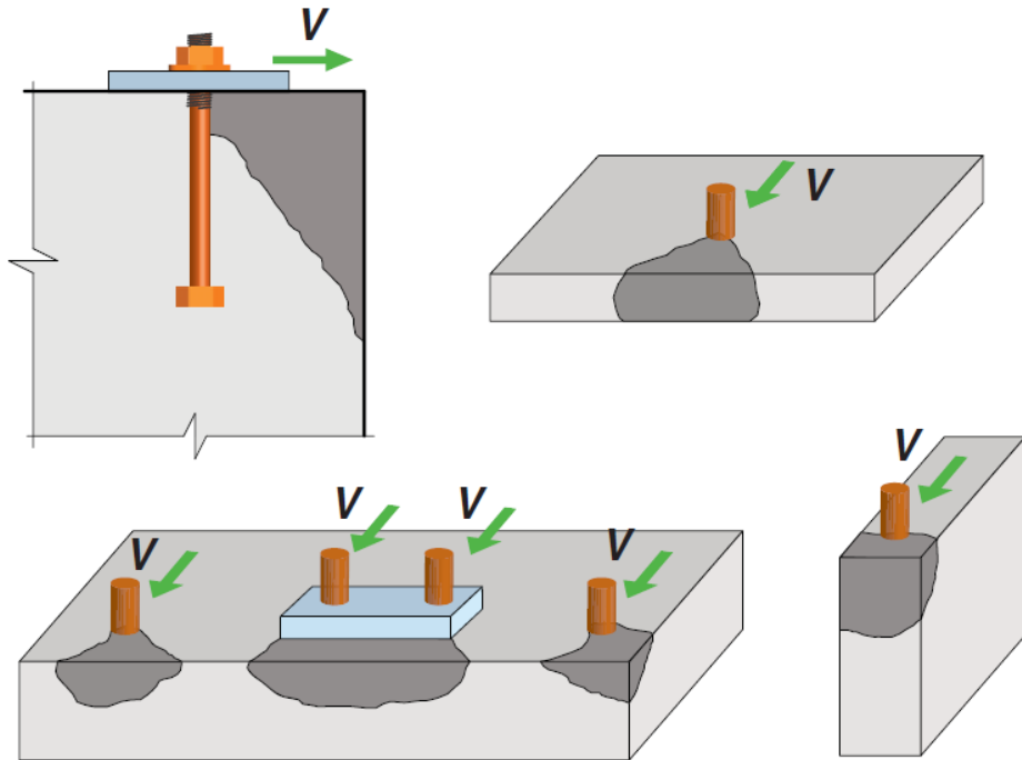
混凝土剪破
