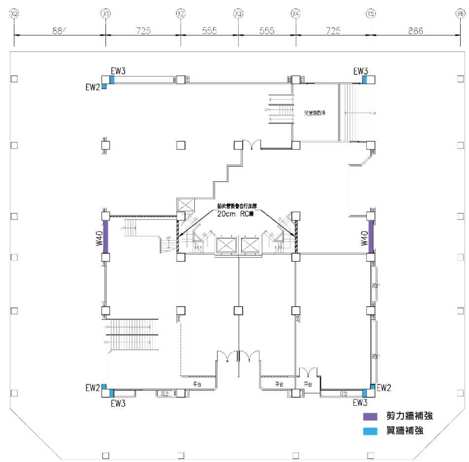
補強平面圖
