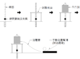
植筋施工之品質
