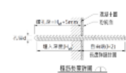
植筋施工之品質
