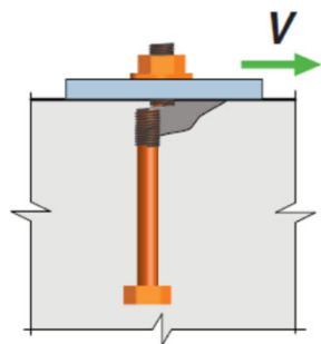
錨栓鋼材剪斷
