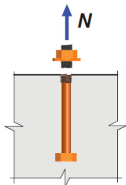
鋼材破壞
