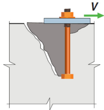
混凝土撬破
