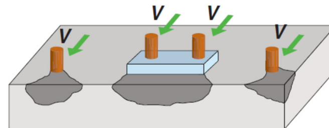
混凝土剪破
