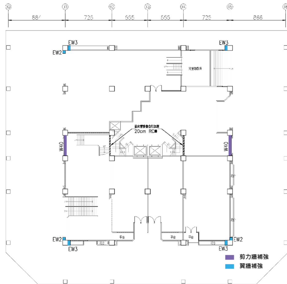
補強平面圖
