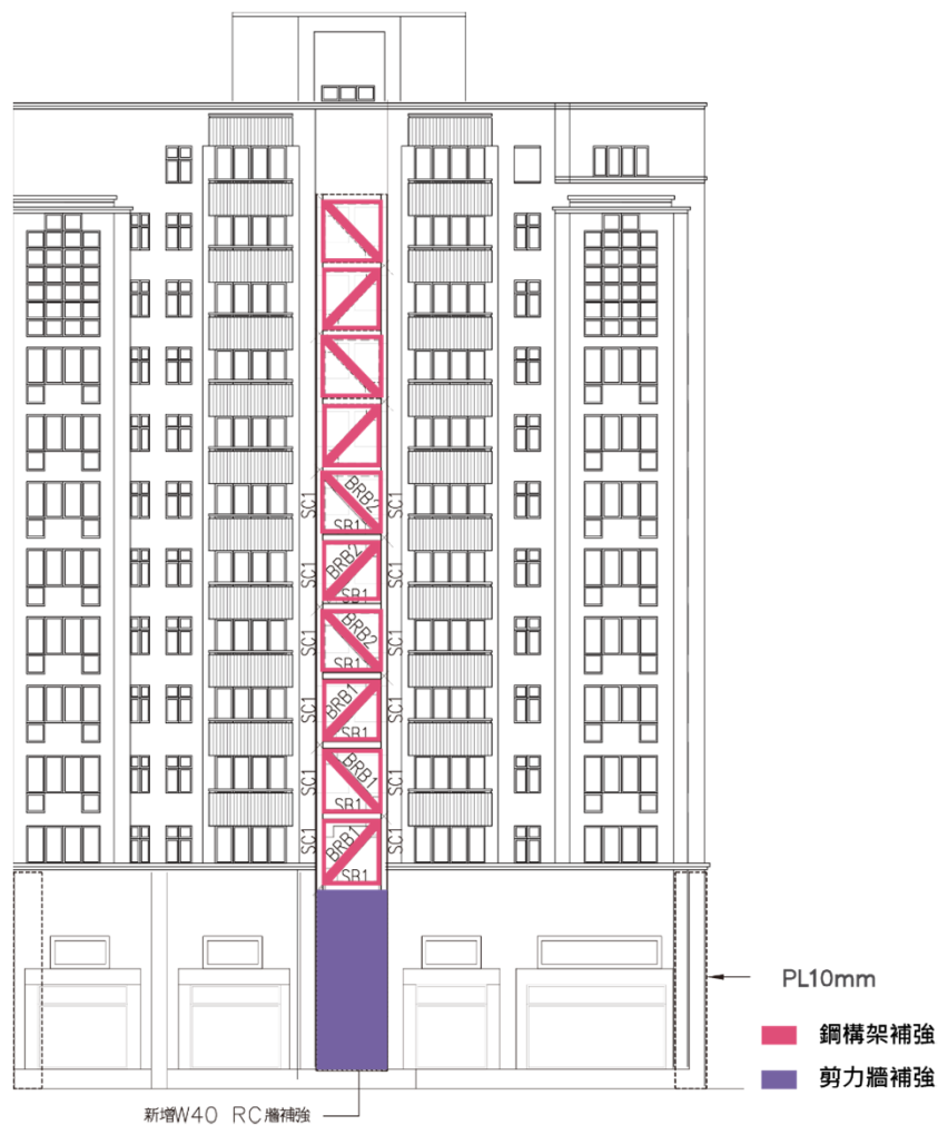
補強立面圖
