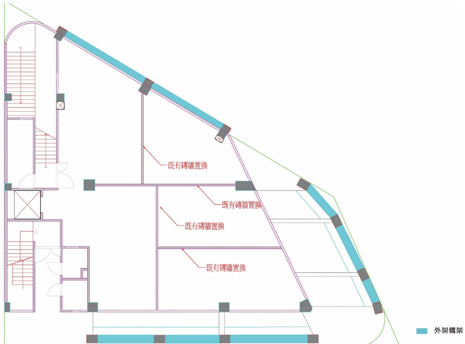
補強位置平面圖
