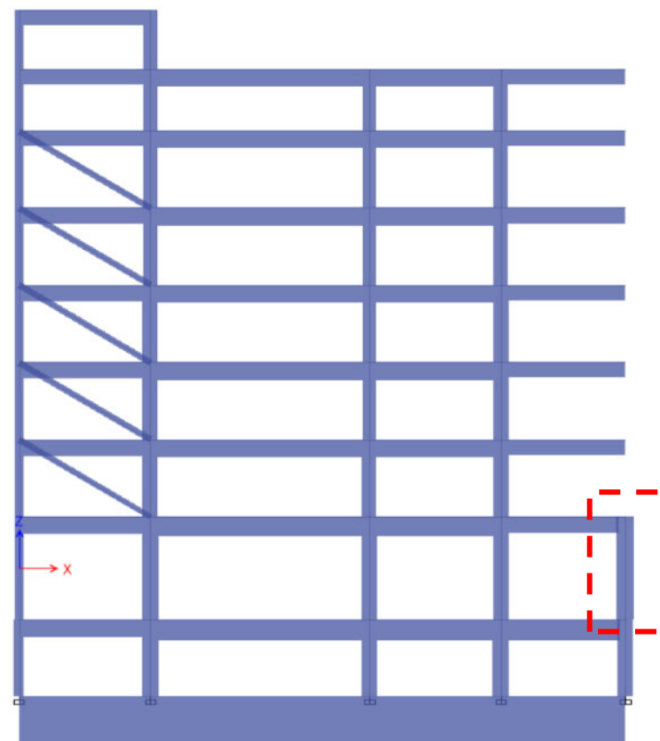
補強後
