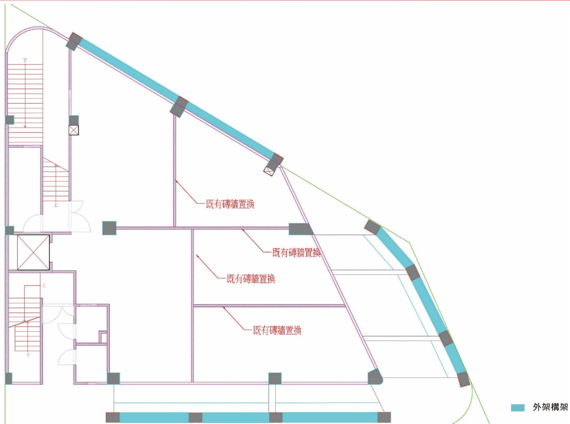
補強位置平面圖
