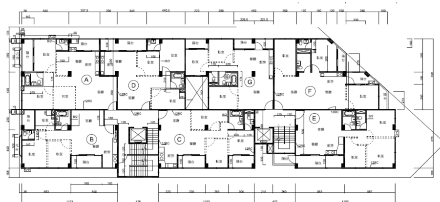
原始2~5F建築平面圖
