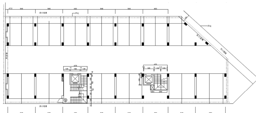
原始1F建築平面圖
