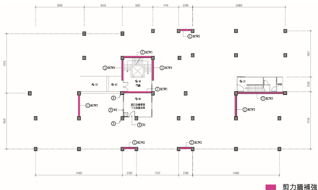
補強位置平面圖
