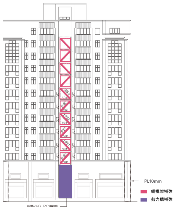
補強立面圖
