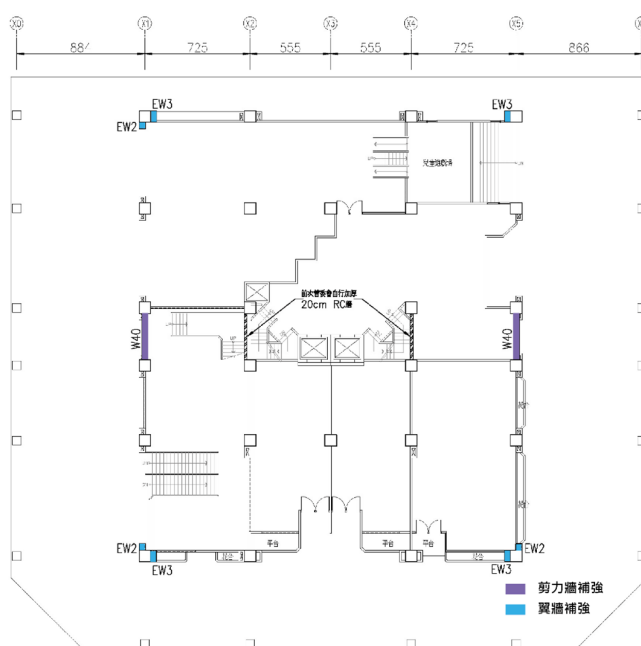
補強平面圖
