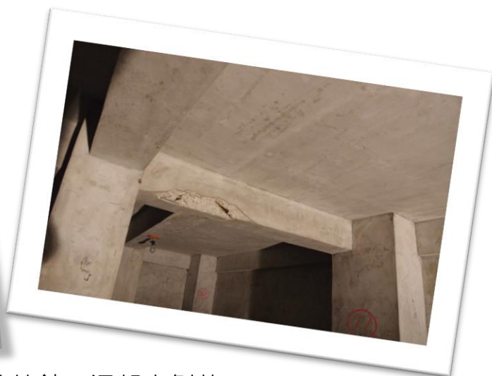
梁柱鋼筋鏽蝕、混凝土剝落
